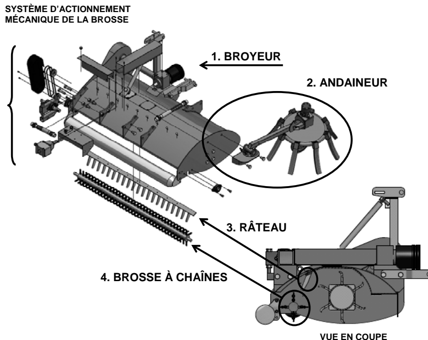
Figure 1 : Les composantes d'un broyeur à litière
