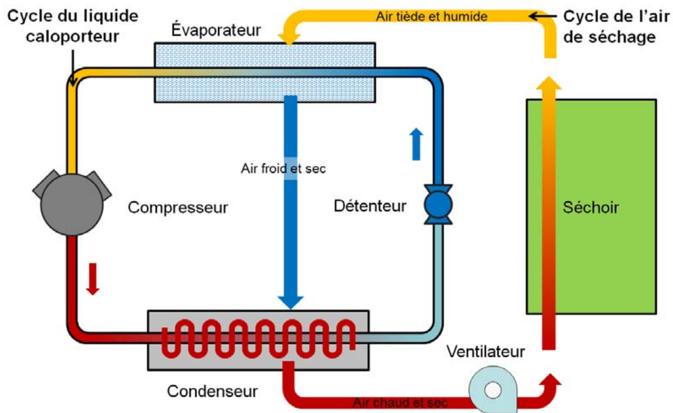
Figure 3. Principe du séchage par déshumidification (source : Agriculture et Agroalimentaire Canada)
