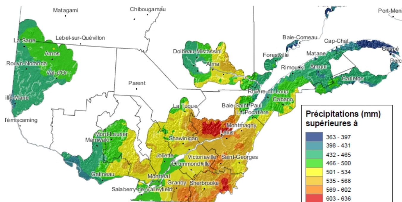
Figure 2. Cumul des précipitations pendant la saison de croissance : probabilité de 8 années sur 10 (source : Atlas agroclimatique, 2012)
